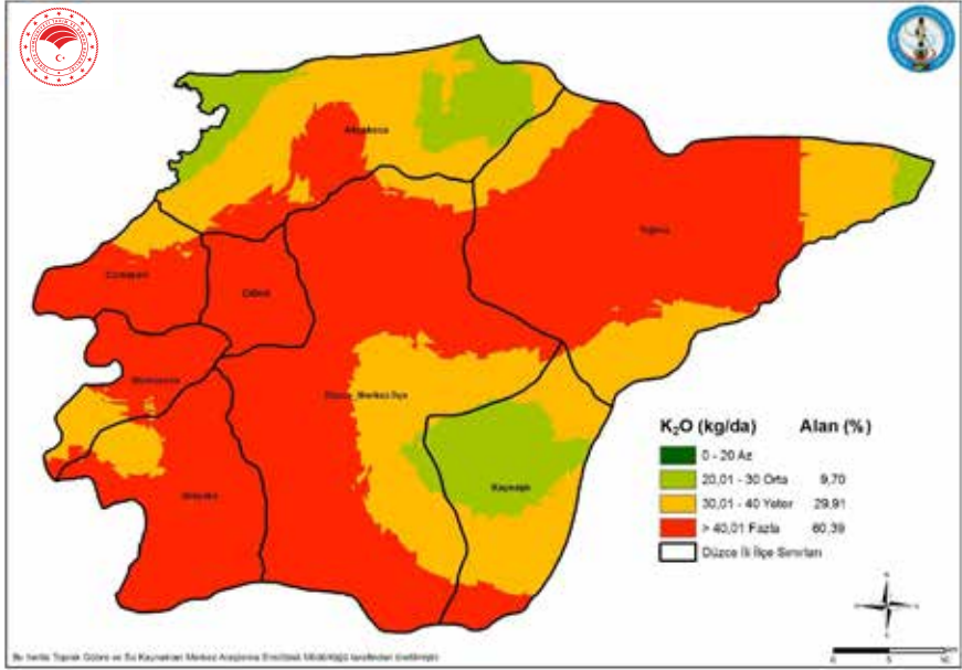
Şekil 3. Düzce İli Topraklarının Potasyum Dağılımları
