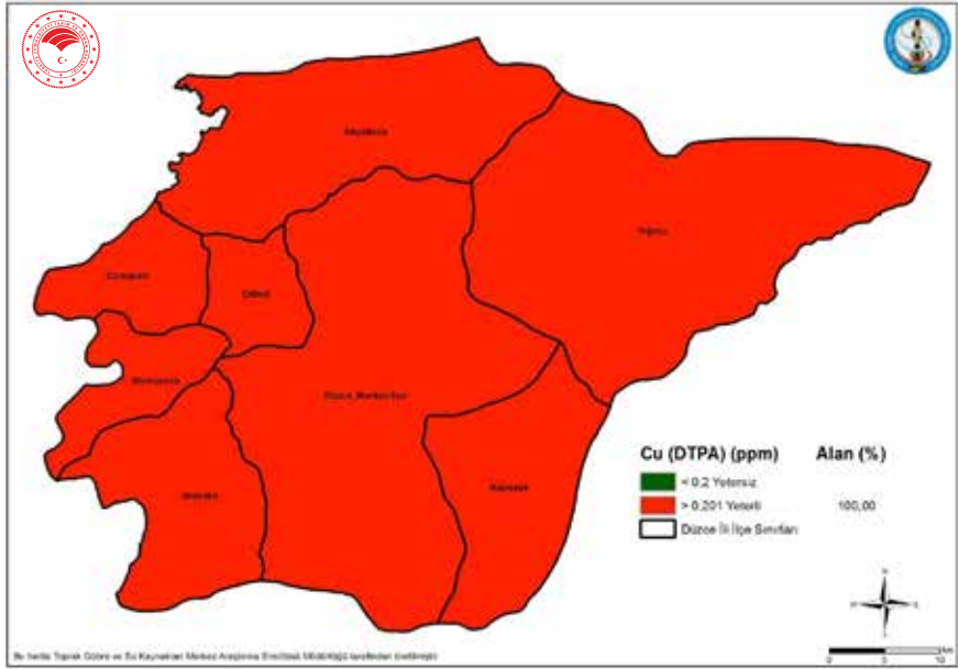
Şekil 5. Düzce İli Topraklarının Bakır Dağılımları
