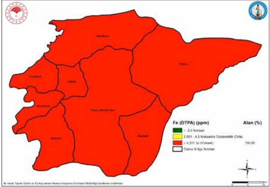
Şekil 4. Düzce İli Topraklarının Demir Dağılımları
