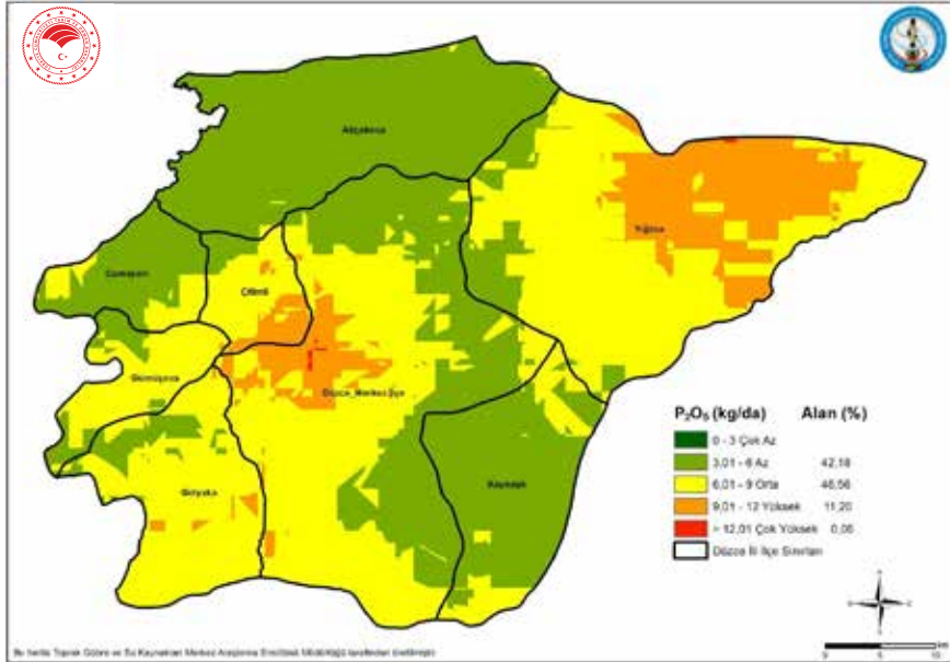
Şekil 2. Düzce İli Topraklarının Fosfor Dağılımları
