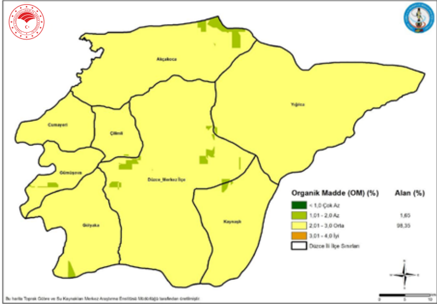
Şekil 1. Düzce İli Topraklarının Organik Madde Dağılımları
