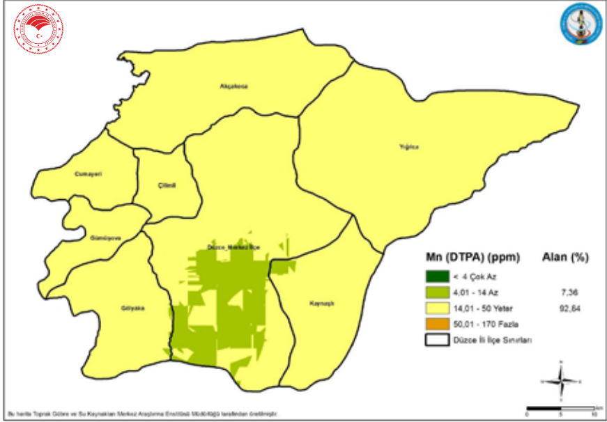
Şekil 7. Düzce İli Topraklarının Mangan Dağılımları
