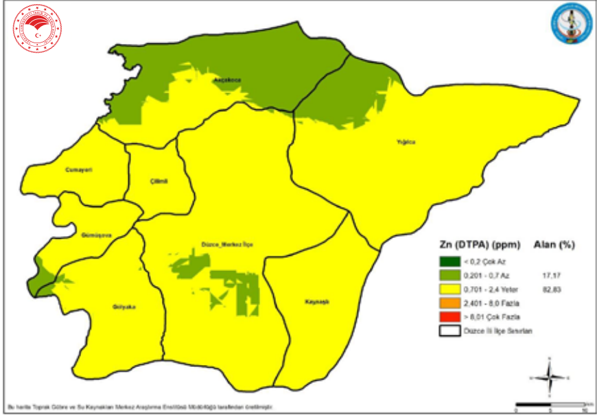
Şekil 6. Düzce İli Topraklarının Çinko Dağılımları
